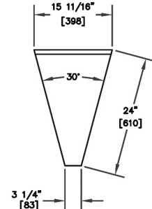
TSF30F-I
