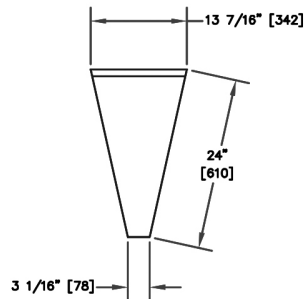
TSF25F-I
