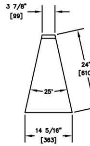
TSF25F-O
