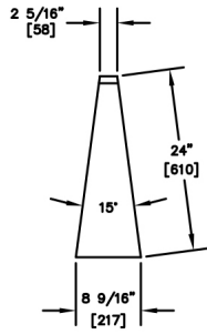
TSF15F-O
