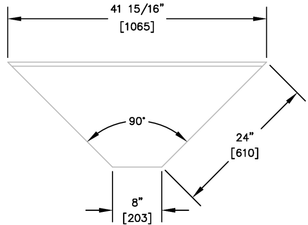
TSF90F-I
