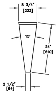
TSF15F-I
