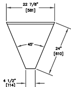
TSF45F-I
