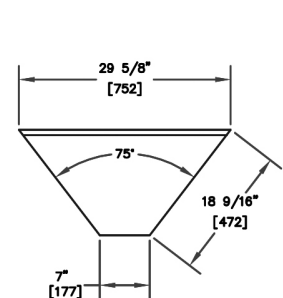
TS75F-I
