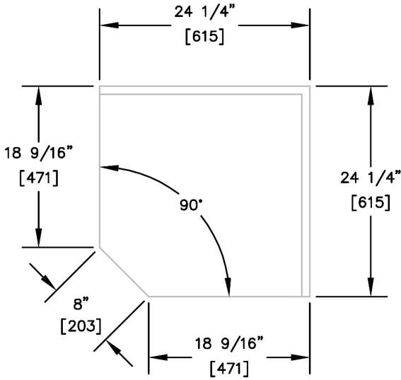
TS90F-FI
