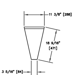
TS25F-I
