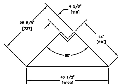
TSF90F-O
