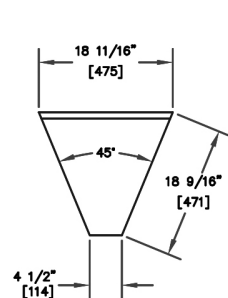
TS45F-I
