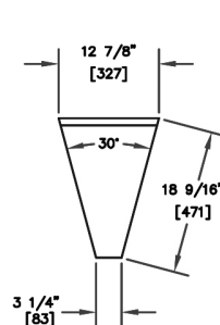
TS30F-I
