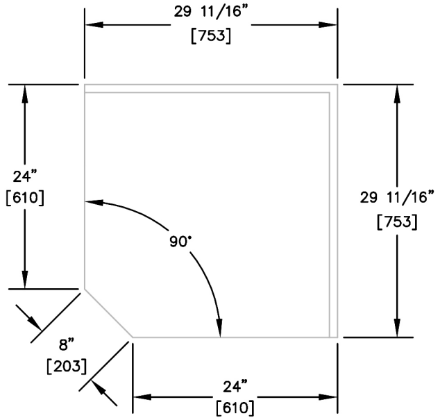
TSF90F-FI
