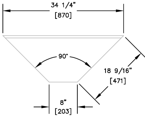
TS90F-I
