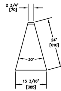
TSF30F-O
