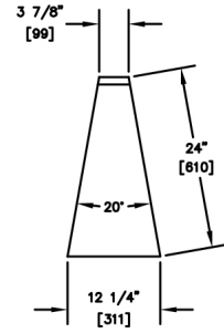
TSF20F-O
