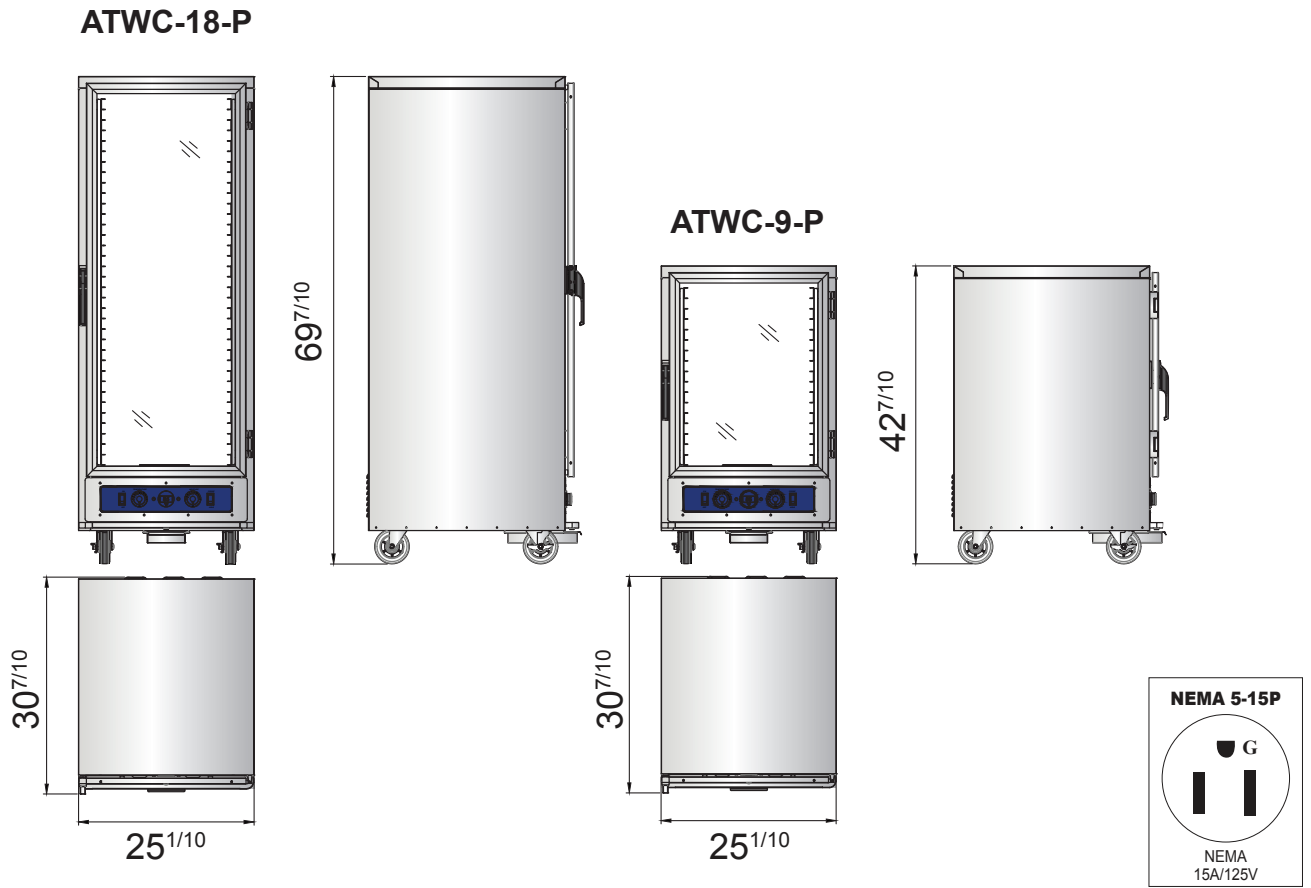
Polycarbonate door
