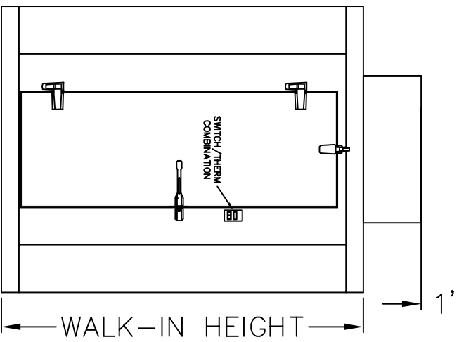
VIEW --A--
