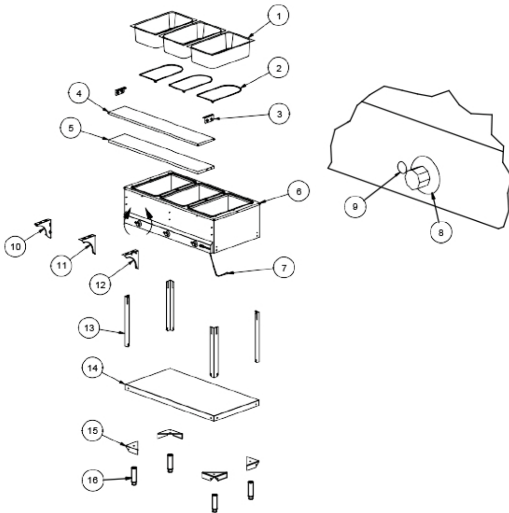
VISTA DETALLADA DE LA LISTA DE PARTES
