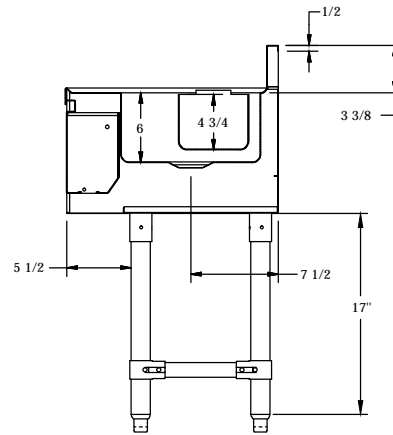
SECTION A-A SCALE 1:12
