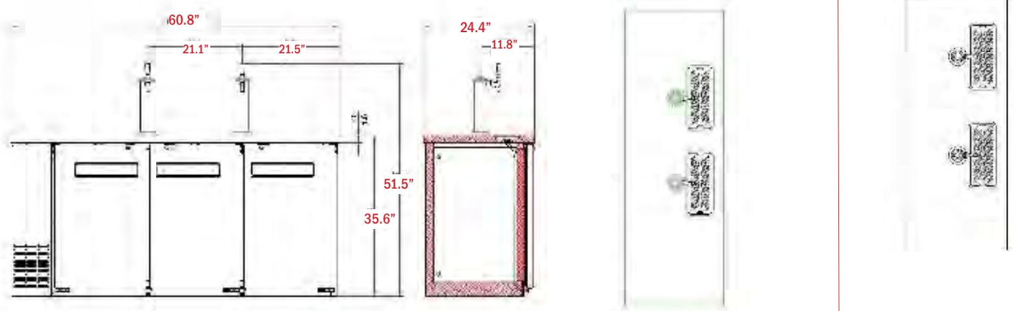
USBD-7224/2
