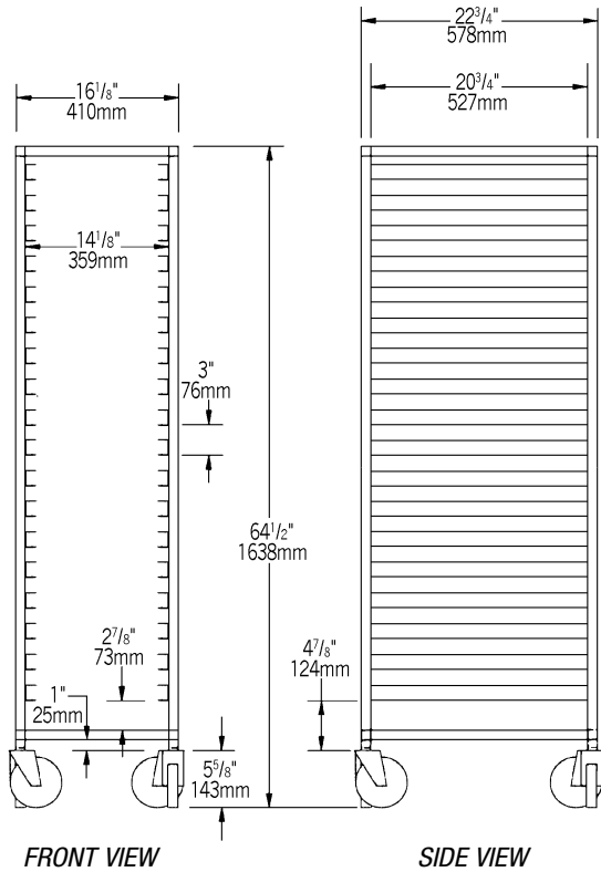
#OUR-1218-3-SR —Single-Width
