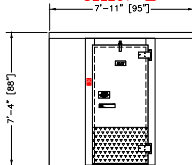
ELEVATION RIGHT HINGE
