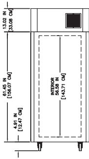
TYP. LEFT END VIEW
